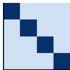
A: equicorrelated
