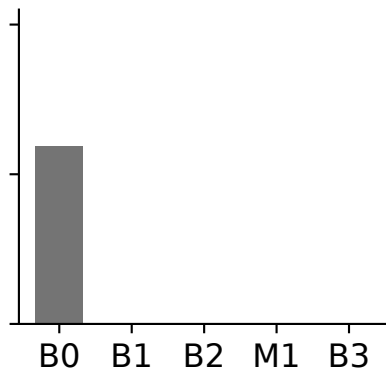
WESAD
