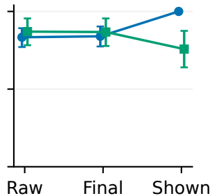
WESAD
