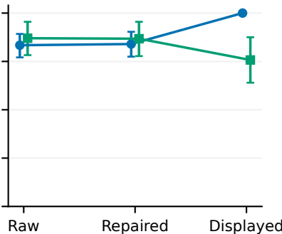
WESAD
