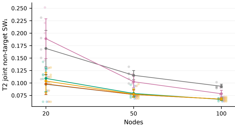
Heteroscedastic
