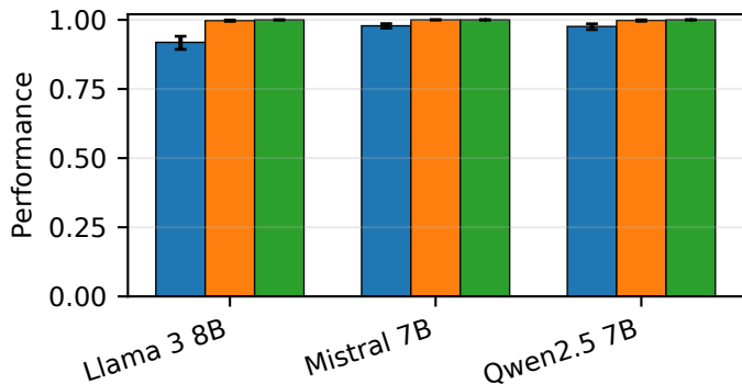
ROC-AUC
