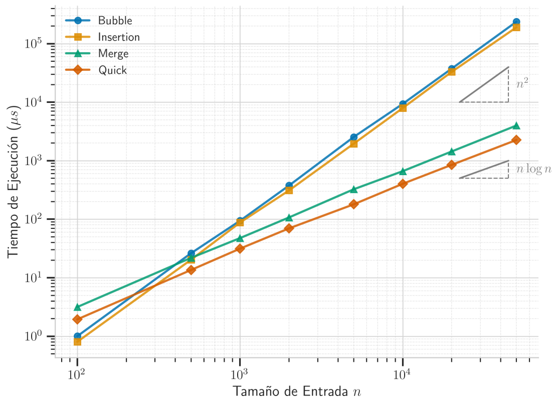
Figura 2: Versión optimizada: escala log-log y marcadores de accesibilidad.
