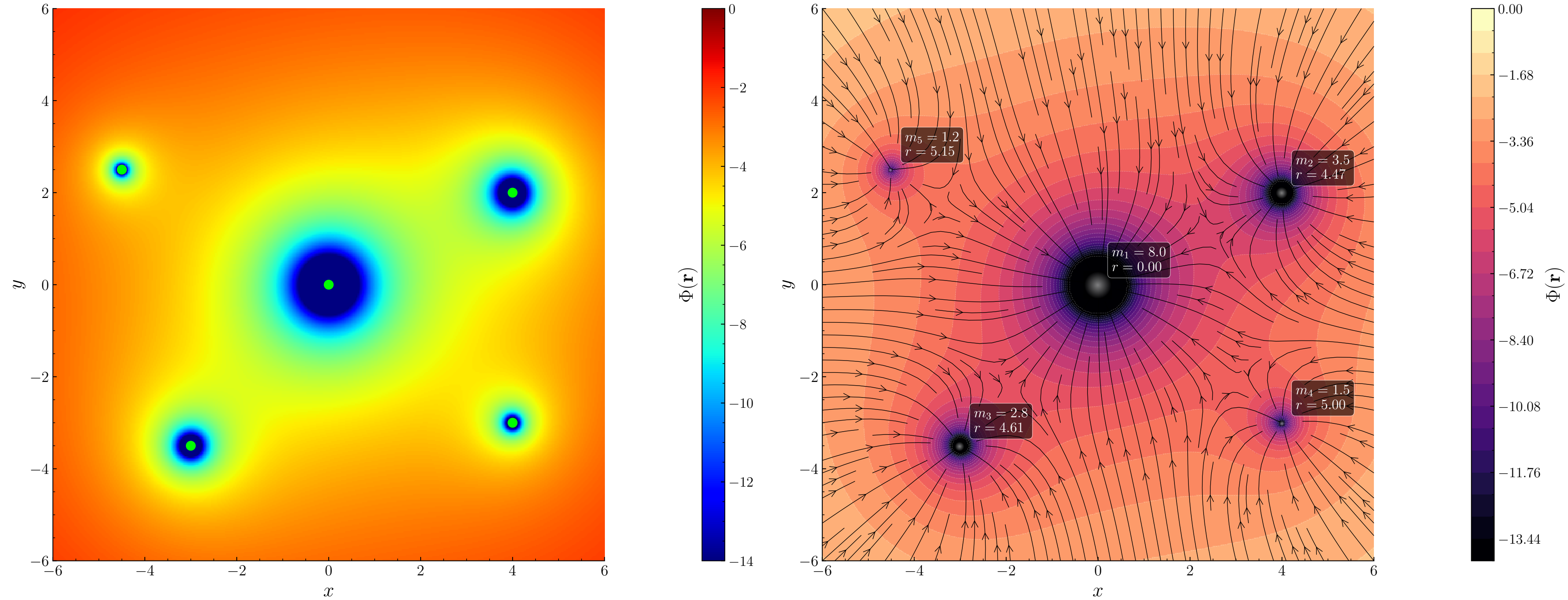
Figura. Potencial gravitacional \Phi(r) para un sistema de N = 5 cuerpos puntuales en escala lineal discreta. Curvas integrales (streamlines) del campo \mathbf{g} = -\nabla\Phi superpuestas. m : masa del cuerpo. r : radio orbital (distancia desde el origen al cuerpo).
