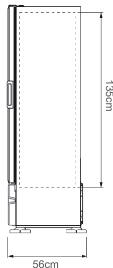
Vista lateral
