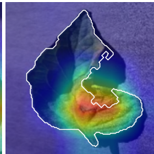
Pred: Tomato tizón tardío (80.9%)
