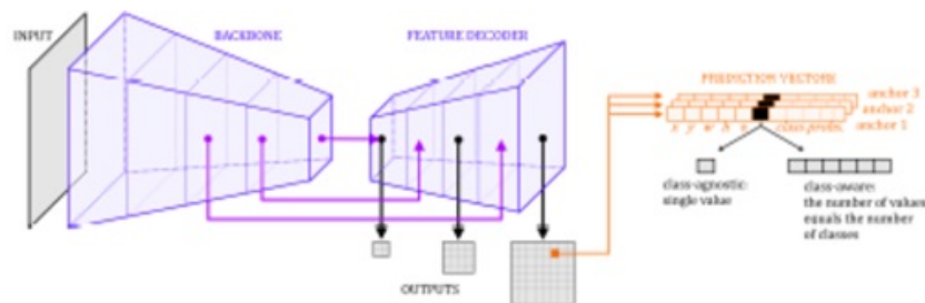
Abbildung 3.3: YOLO-Architektur
