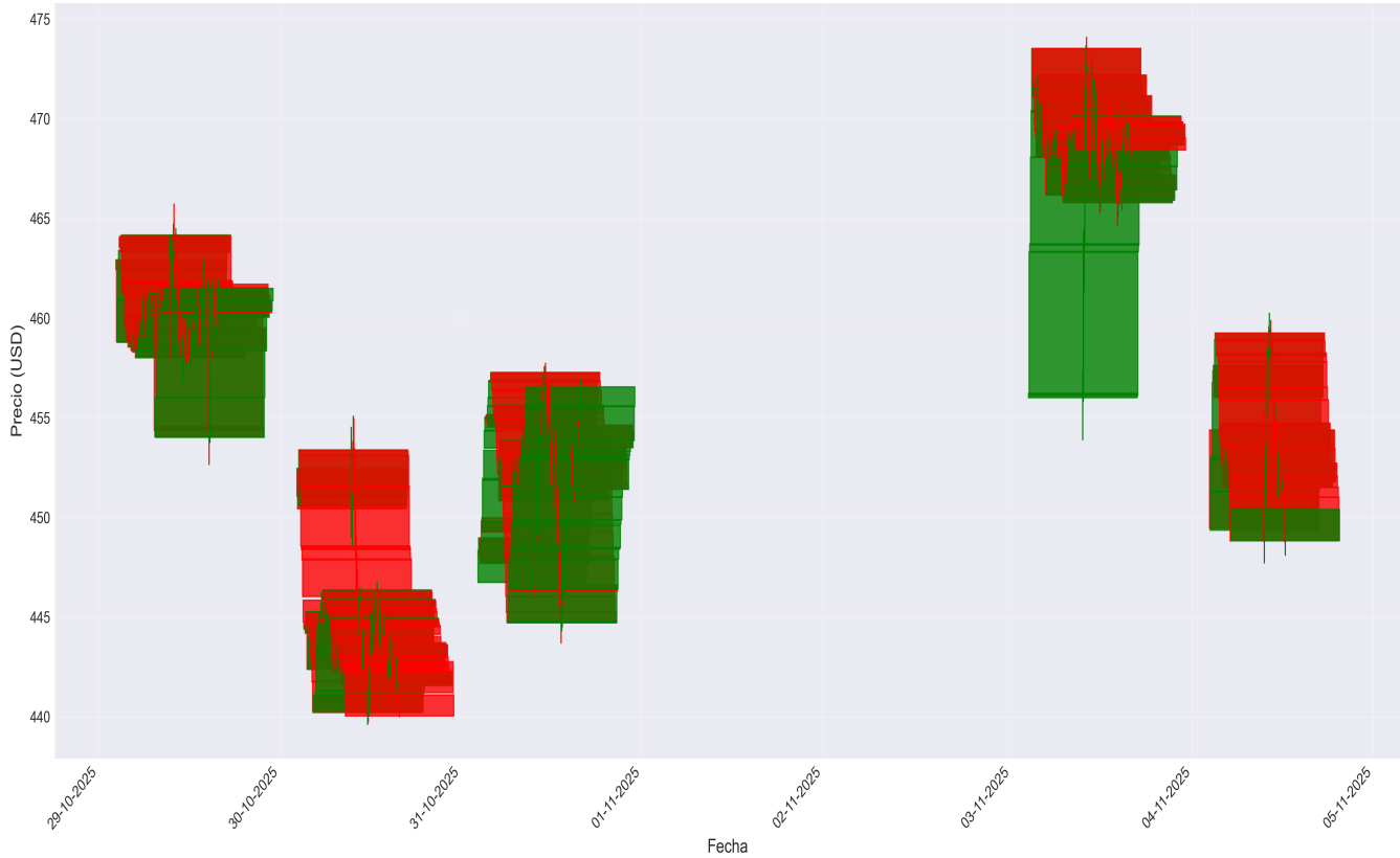
Gráfico de Velas: Tesla
