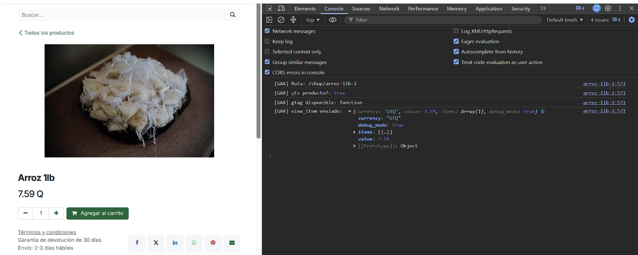
Figura 3. Validación del evento view_item en la ficha Arroz 1lb mediante la consola del navegador.
