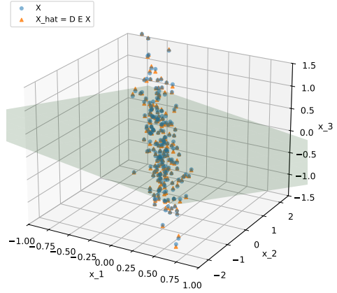
Original X (azul) vs. reconstrucción \hat{X} (naranja) Subespacio aprendido en verde
