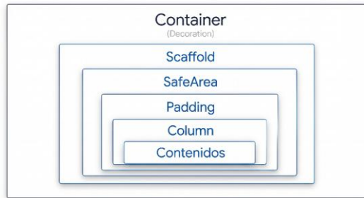
Figura 20 - Esquema de anidación: PantallaContenidos.
