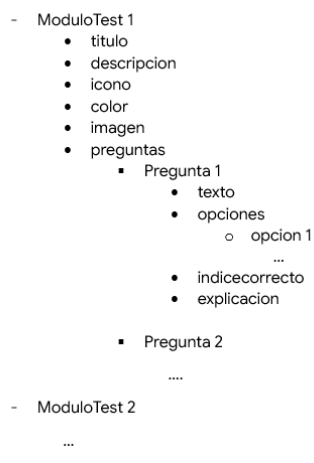
Figura 30 - Esquema de la estructura de la base de datos local de "tests.dart"
