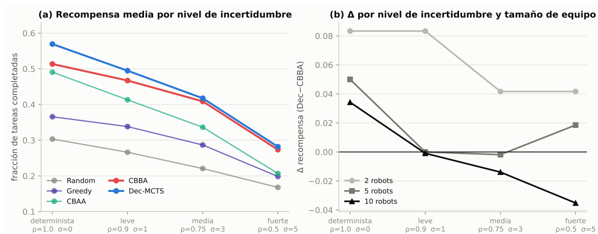
Figura 6.6: Bloque E. En (a), recompensa media de los cinco algoritmos en cada uno de los cuatro niveles del gradiente de incertidumbre. En (b), diferencia pareada \Delta en esos mismos niveles, desglosada por tamaño de equipo. Cada nivel del gradiente reúne 18 escenarios.
