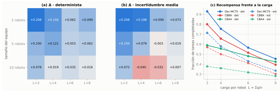
Figura 6.5: Bloque C. Diferencia pareada \Delta en la rejilla de tamaño de equipo \times carga por robot, en régimen determinista (a) y con incertidumbre media (b): el azul señala \Delta > 0 y el rojo \Delta < 0 , con intensidad proporcional a la magnitud. La columna L = 6 corresponde al control del bloque A. El panel (c) recoge la recompensa media de los tres algoritmos coordinados frente a la carga.
