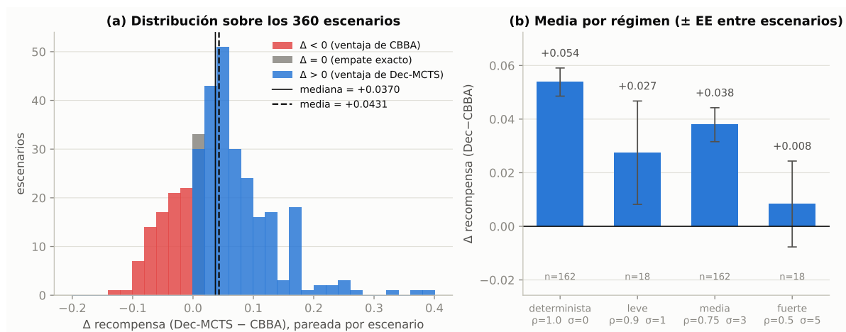
Figura 6.2: Diferencia pareada \Delta entre Dec-MCTS y CBBA. En (a), su distribución sobre los 360 escenarios: cada escenario aporta una observación, coloreada según el signo de la diferencia; la línea continua marca la mediana y la discontinua, la media. En (b), la media por régimen de incertidumbre con su error estándar entre escenarios; los regímenes lev y fue proceden únicamente del bloque E, de ahí su menor número de escenarios y su mayor variabilidad.
