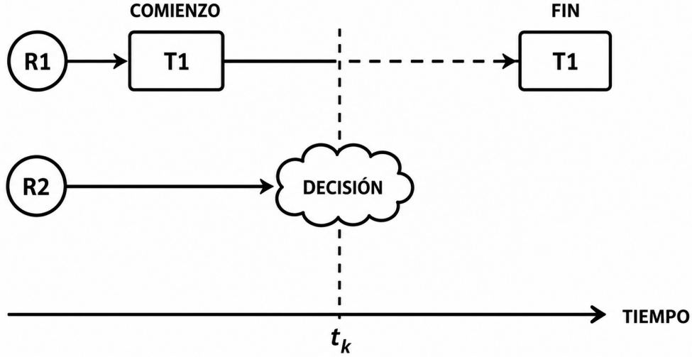
Figura 2.2: Ilustración del leak temporal . En el instante t_k , el robot R_2 debe decidir su siguiente acción mientras R_1 ejecuta la tarea T_1 , comenzada con anterioridad. Sin embargo, el instante de finalización de T_1 (el evento FIN, aún no producido) ya se ha muestreado y guardado en el estado al COMIENZO de la tarea, la decisión de R_2 podría depender de información futura que no estaría disponible en una ejecución real.
