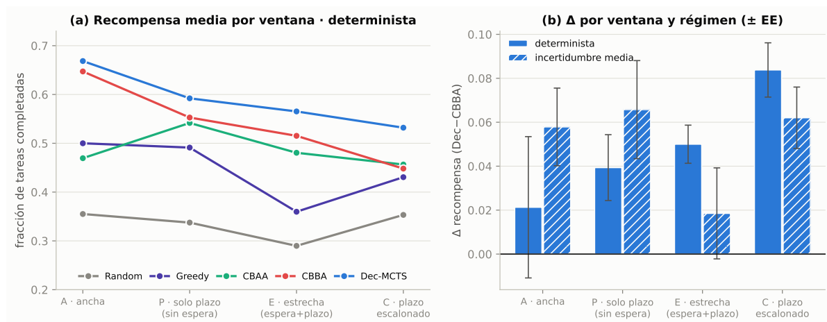
Figura 6.4: Bloque B. En (a), recompensa media de los cinco algoritmos en régimen determinista para cada forma de ventana. En (b), diferencia pareada \Delta en esas mismas ventanas, en los dos regímenes y con su error estándar entre escenarios.
