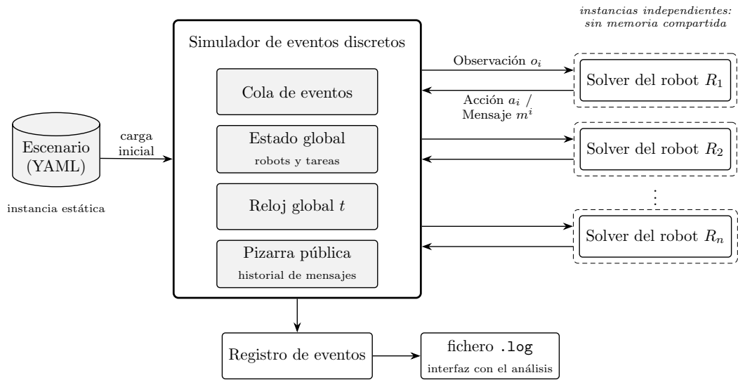
Figura 4.1: Arquitectura del simulador distribuido y flujo de datos entre sus componentes. Cada robot dispone de una instancia independiente de solver; la única información que cruza de un robot a otro es la comunicación de mensajes.
