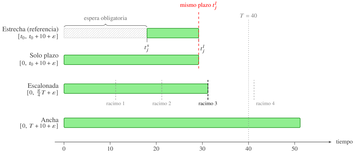
Figura 5.2: Las cuatro tipologías de ventana de ejecución, derivadas de los mismos sorteos t_0 y \varepsilon para una misma tarea, perteneciente en el ejemplo al tercer racimo. La ventana estrecha y la de solo plazo cierran exactamente en el mismo instante y difieren únicamente en la espera obligatoria que impone la primera, lo que aísla la espera como factor. En la escalonada el plazo depende del racimo: las marcas discontinuas señalan los cuatro cierres posibles y la destacada es la que corresponde a la tarea representada. La ventana ancha no impone acoplamiento temporal alguno.
