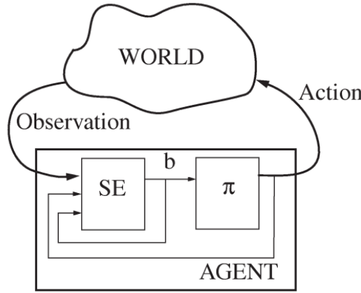
Figura 2.1: En un POMDP, un agente se puede descomponer en un estimador de estado (SE) y una política ( \pi ).
