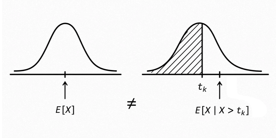
Figura 2.3: La duración de una tarea no es, en general, sin memoria. La esperanza incondicional \mathbb{E}[X] (izquierda) difiere de la esperanza condicionada a que la tarea siga en ejecución transcurrido un tiempo t_k , \mathbb{E}[X \mid X > t_k] (derecha): el tiempo ya transcurrido desplaza la distribución del tiempo restante.
