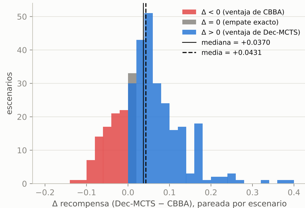
(a) Distribución sobre los 360 escenarios
