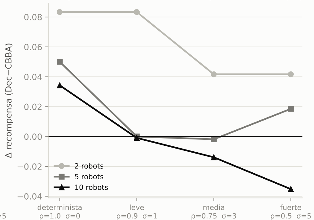
(b) \Delta por nivel de incertidumbre y tamaño de equipo
