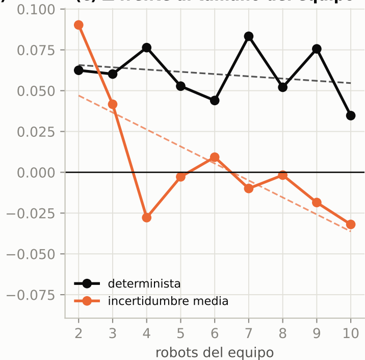
(c) \Delta frente al tamaño del equipo
