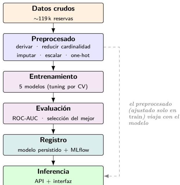
Figura 10: El pipeline de ML de extremo a extremo (flujo vertical): preprocesado, entrenamiento y evaluación de los modelos, registro del ganador e inferencia. El preprocesado se aprende del entrenamiento y se persiste junto al modelo, de modo que predecir reproduce exactamente las transformaciones del entrenamiento.
