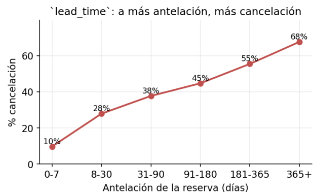
Figura 5: Tasa de cancelación por tramos de lead_time : relación creciente y casi monótona, la señal numérica más fuerte.
