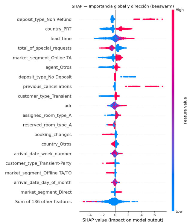
Figura 10: Resumen SHAP global ( beeswarm ) del modelo ganador: aporte de cada variable a la predicción. Confirma los hallazgos del EDA.
