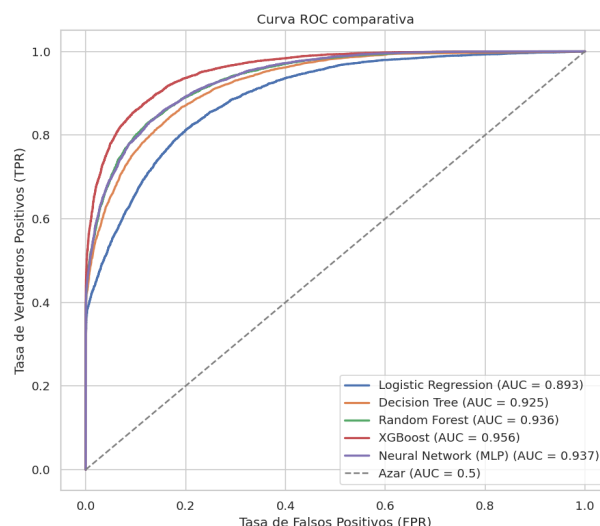
Figura 13: Curvas ROC comparativas. Cuanto más cerca de la esquina superior izquierda, mejor; XGBoost domina al resto.
