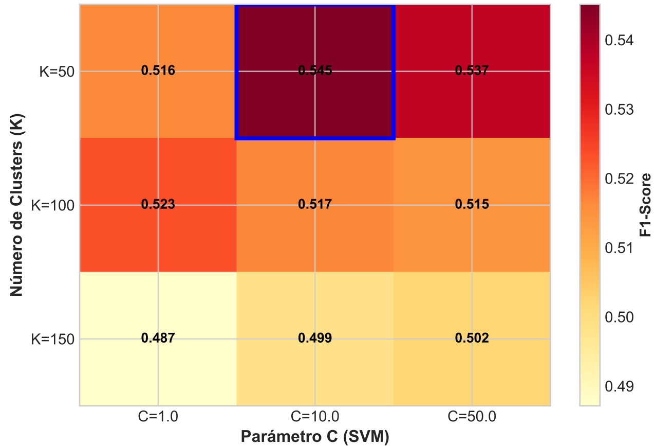
Grid Search: F1-Score por Combinación de Hiperparámetros
