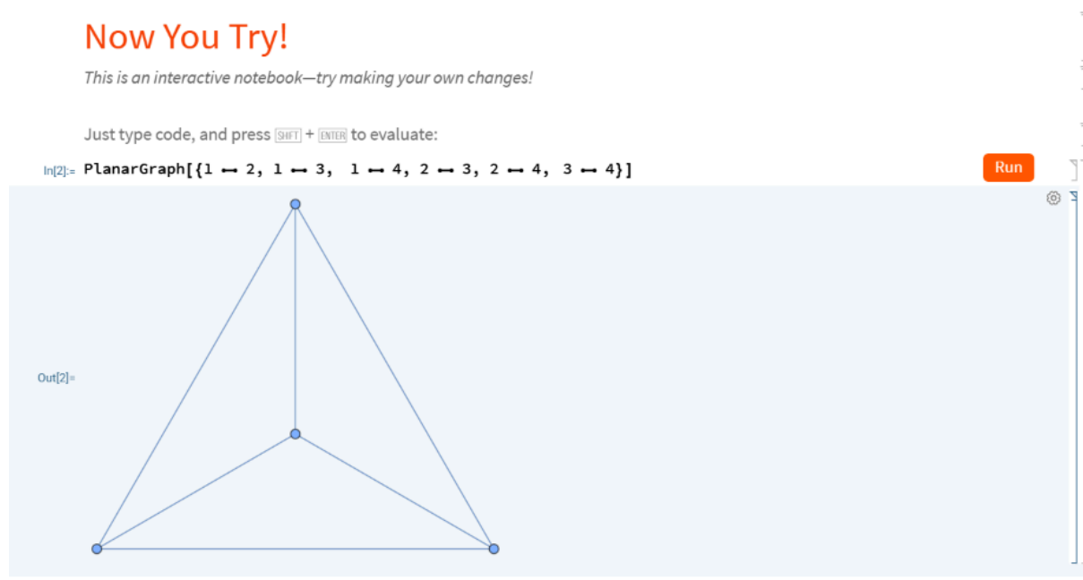
Figure 1: 実行例
