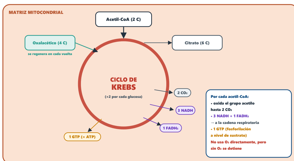
Figura 3. Entradas y salidas de una vuelta del ciclo de Krebs.
