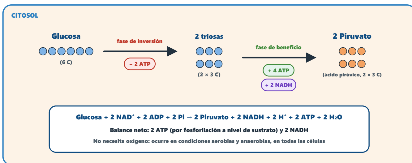
Figura 1. Visión global de la glucólisis (sin intermediarios).
