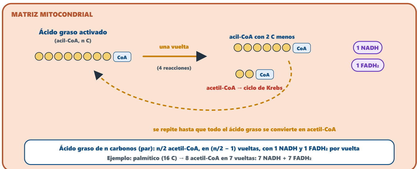
Figura 5. La \beta -oxidación separa el ácido graso en unidades de dos carbonos.
