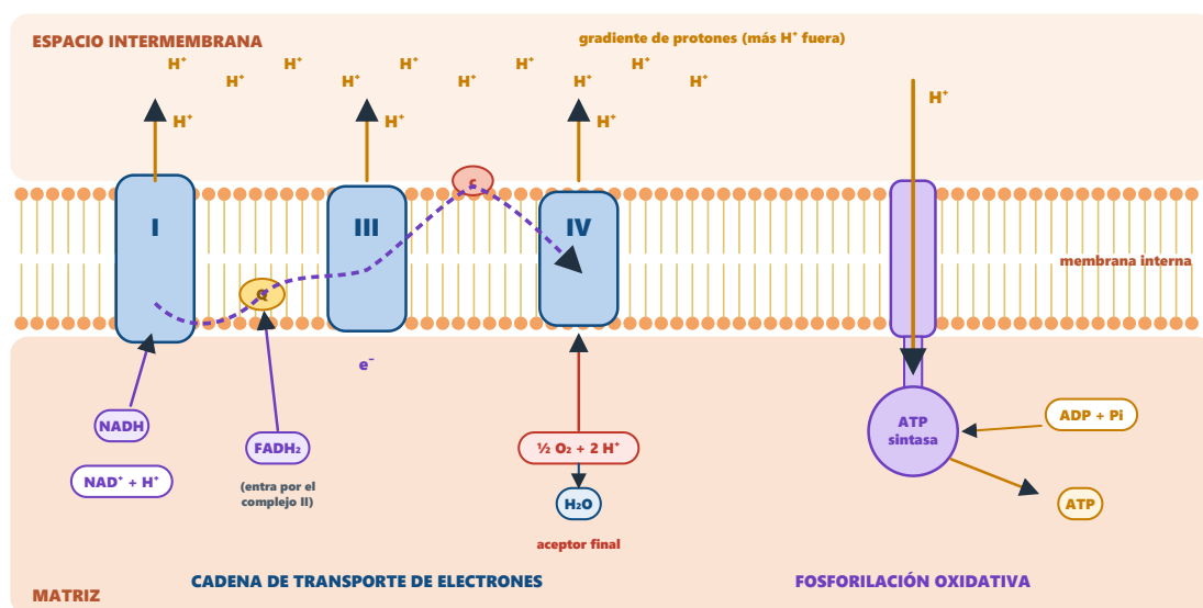
Figura 4. Cadena de transporte de electrones y fosforilación oxidativa (como en el modelo de examen de 2026).
