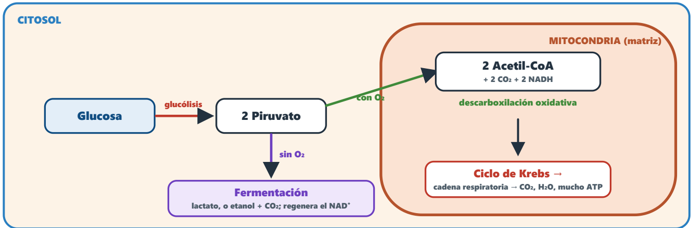
Figura 2. El oxígeno decide el camino del piruvato.
