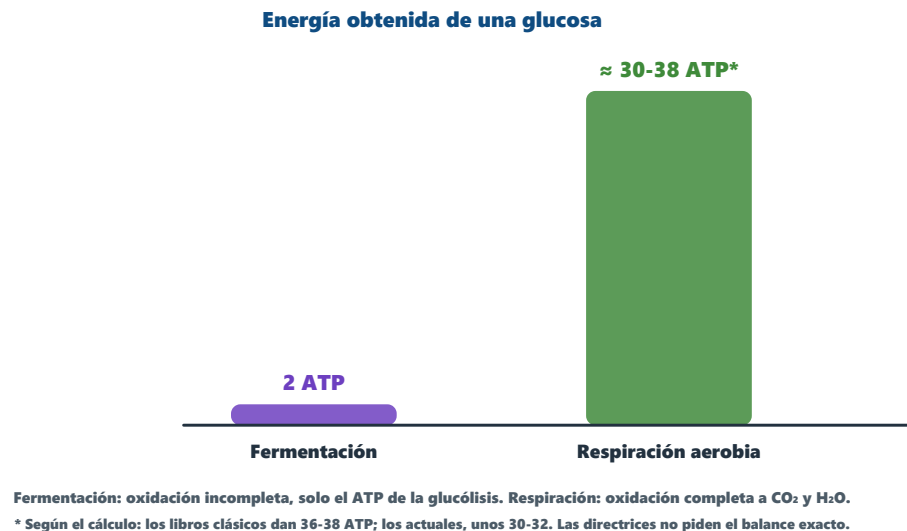
Figura 6. La respiración rinde muchísimo más que la fermentación.
