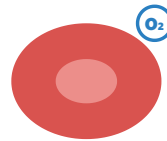
Transporte hemoglobina
