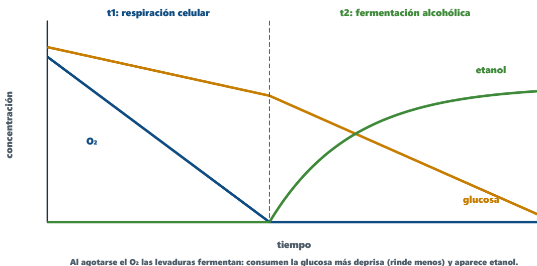
Figura 2. Levaduras en un recipiente cerrado (como en las preguntas de 2015 y 2022).
