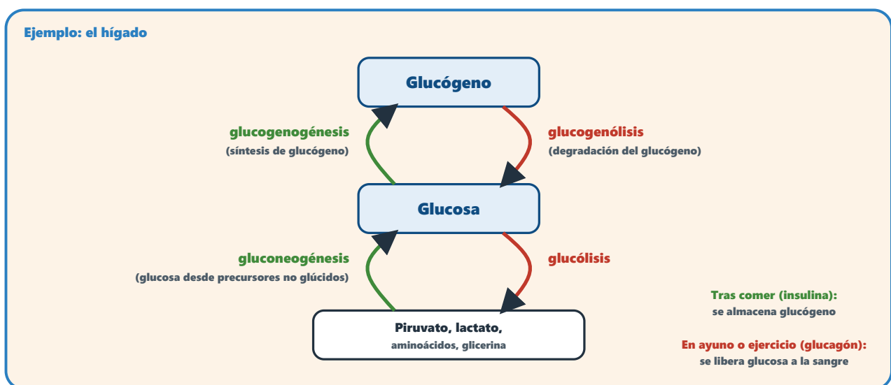
Figura 2. Síntesis y degradación del glucógeno y de la glucosa.
