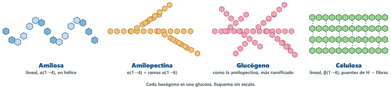
Figura 8. Los homopolisacáridos de glucosa (esquema sin escala).
