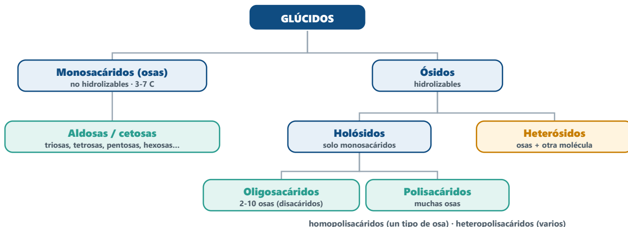
Figura 1. Clasificación de los glúcidos.
