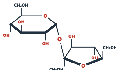
Figura 7. Los cuatro disacáridos de las directrices (se omiten los H).
