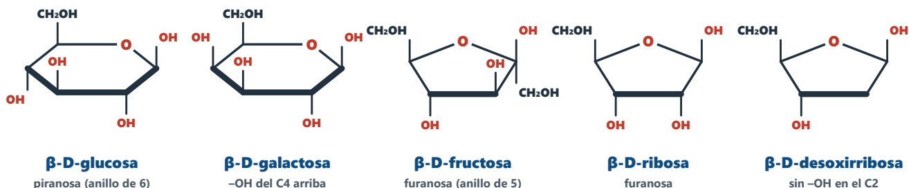
Figura 5. Formas cíclicas β de los monosacáridos de las directrices.
