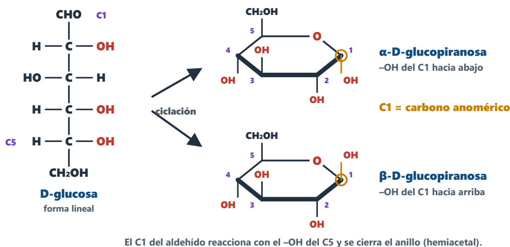
Figura 4. Ciclación de la glucosa en proyección de Haworth (se omiten los H).
