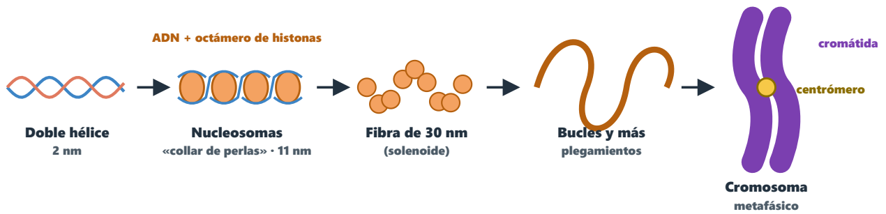
Figura 6. Del ADN al cromosoma (esquema sin escala).
