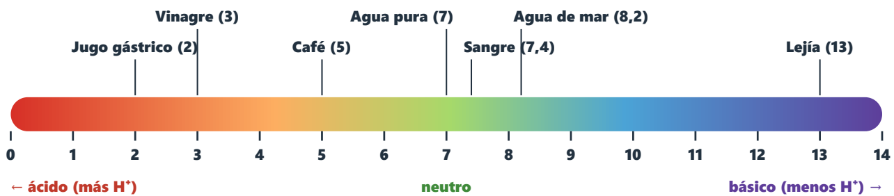
Figura 14. La escala de pH.
