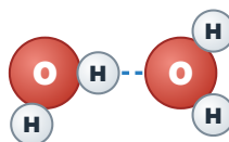
Puente de hidrógeno entre H ( \delta^+ ) y O o N ( \delta^- )
