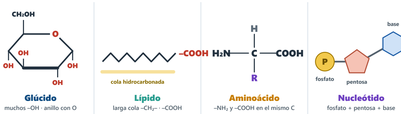
Figura 3. Las «señas de identidad» de cada tipo de biomolécula.
