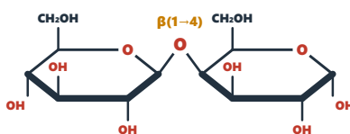
Celobiosa
