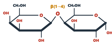
Lactosa
