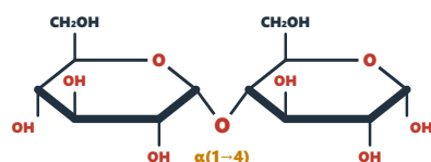
Maltosa
