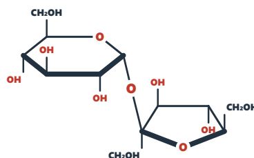
Celobiosa
