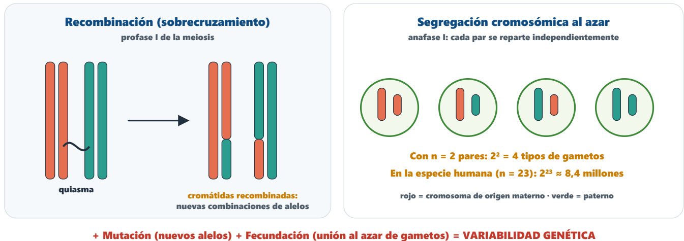
Figura 6. Fuentes de variabilidad genética.
