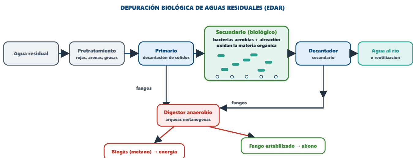
Figura 7. Una estación depuradora de aguas residuales (EDAR).
