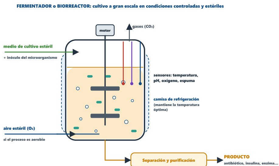
Figura 2. Un fermentador o biorreactor: el microorganismo crece en condiciones óptimas y controladas.
