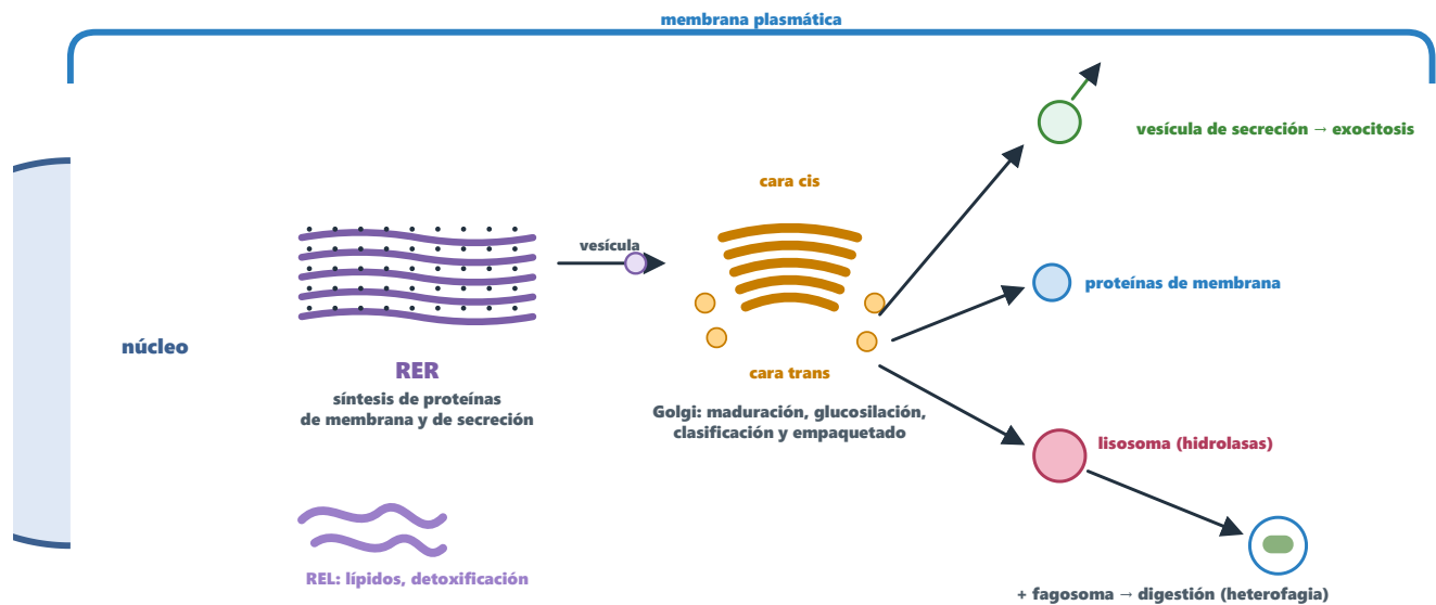
Figura 12. Ruta de las proteínas en el sistema de endomembranas.
