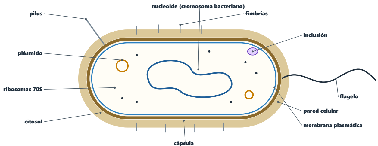
Figura 5. Componentes de una bacteria.
