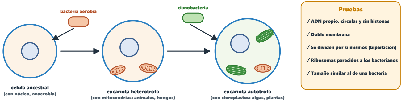
Figura 15. Origen endosimbiótico de mitocondrias y cloroplastos (Lynn Margulis, 1967).
