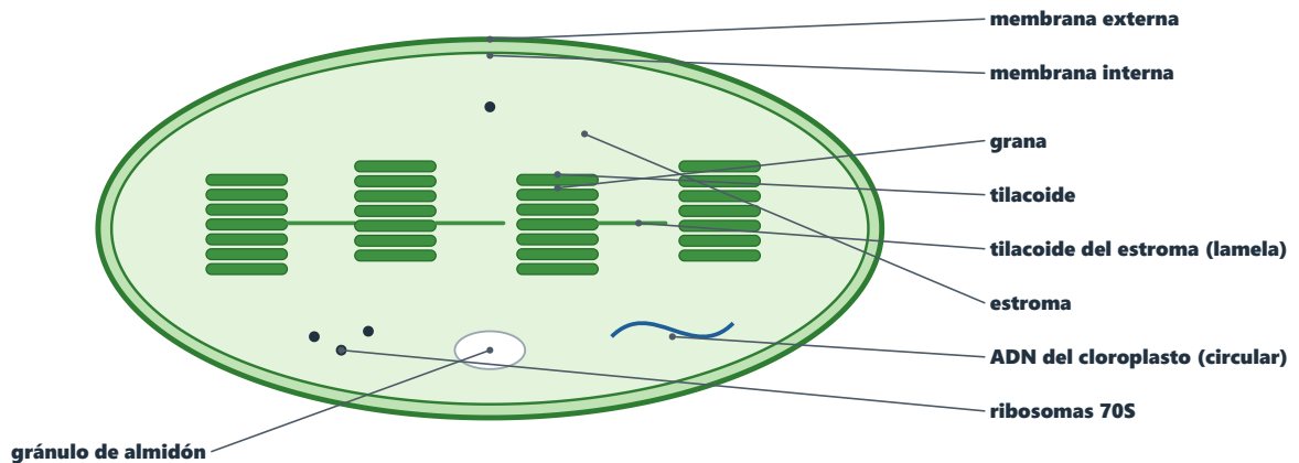
Figura 14. Estructura del cloroplasto.
