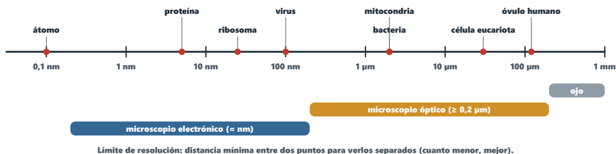
Figura 2. Tamaños y qué instrumento permite verlos.
