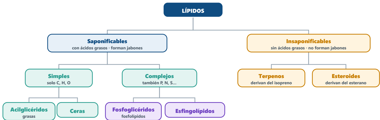
Figura 2. Clasificación de los lípidos.
