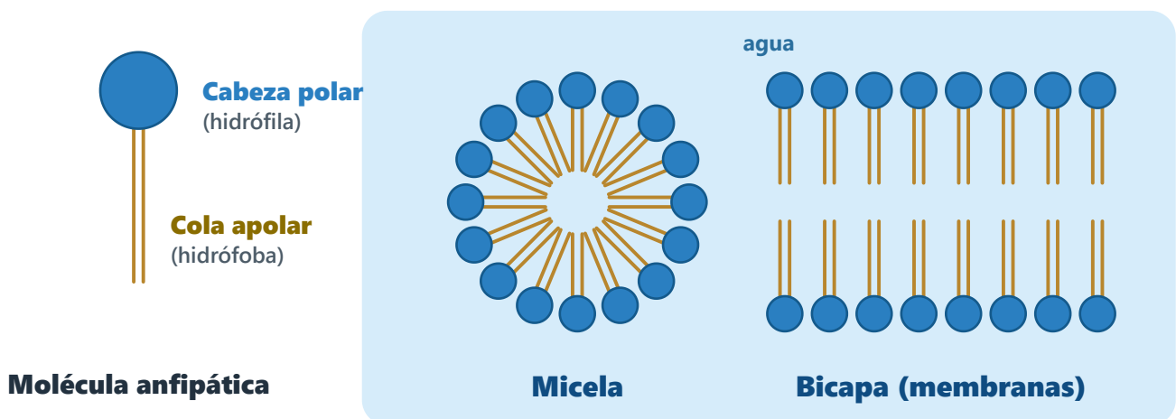
Figura 9. Organización de los lípidos anfipáticos en el agua.
