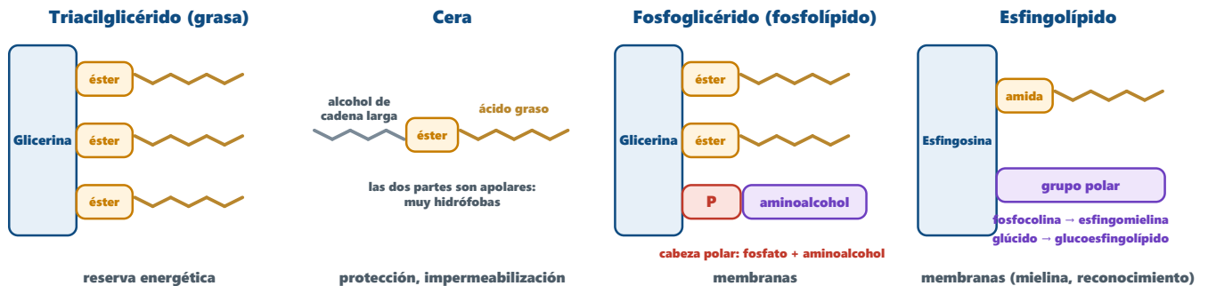
Figura 7. Composición de los lípidos saponificables.
