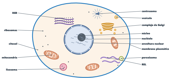
Figura 3. Célula eucariota animal.
