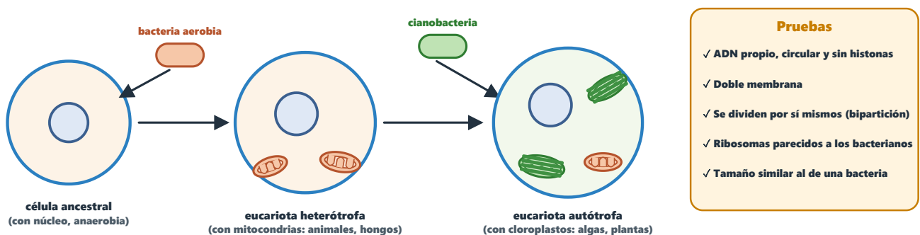
Figura 15. Origen endosimbiótico de mitocondrias y cloroplastos (Lynn Margulis, 1967).
