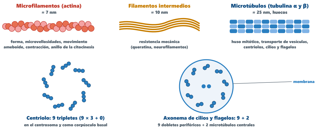
Figura 10. Componentes del citoesqueleto y estructuras formadas por microtubulos.
