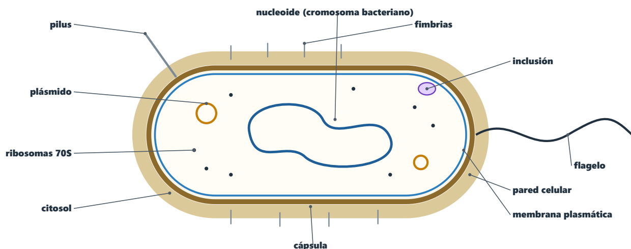
Figura 5. Componentes de una bacteria.
