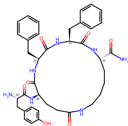
ZH831 (714 Da)
