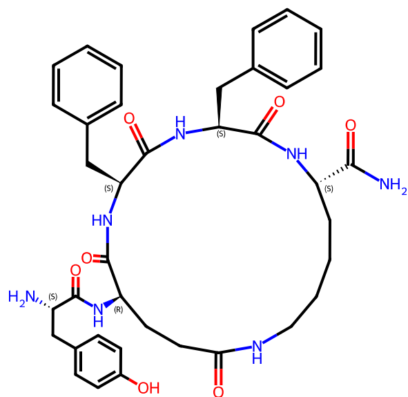
ZH831 (714 Da)
