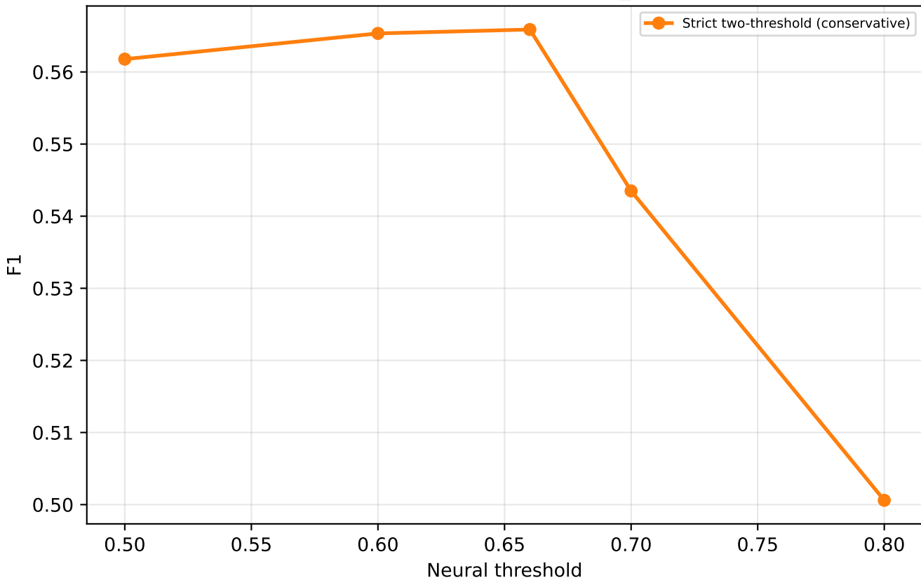
F1 vs threshold — strict conservative \tau_{\text{high}}=0.80 (valid)
