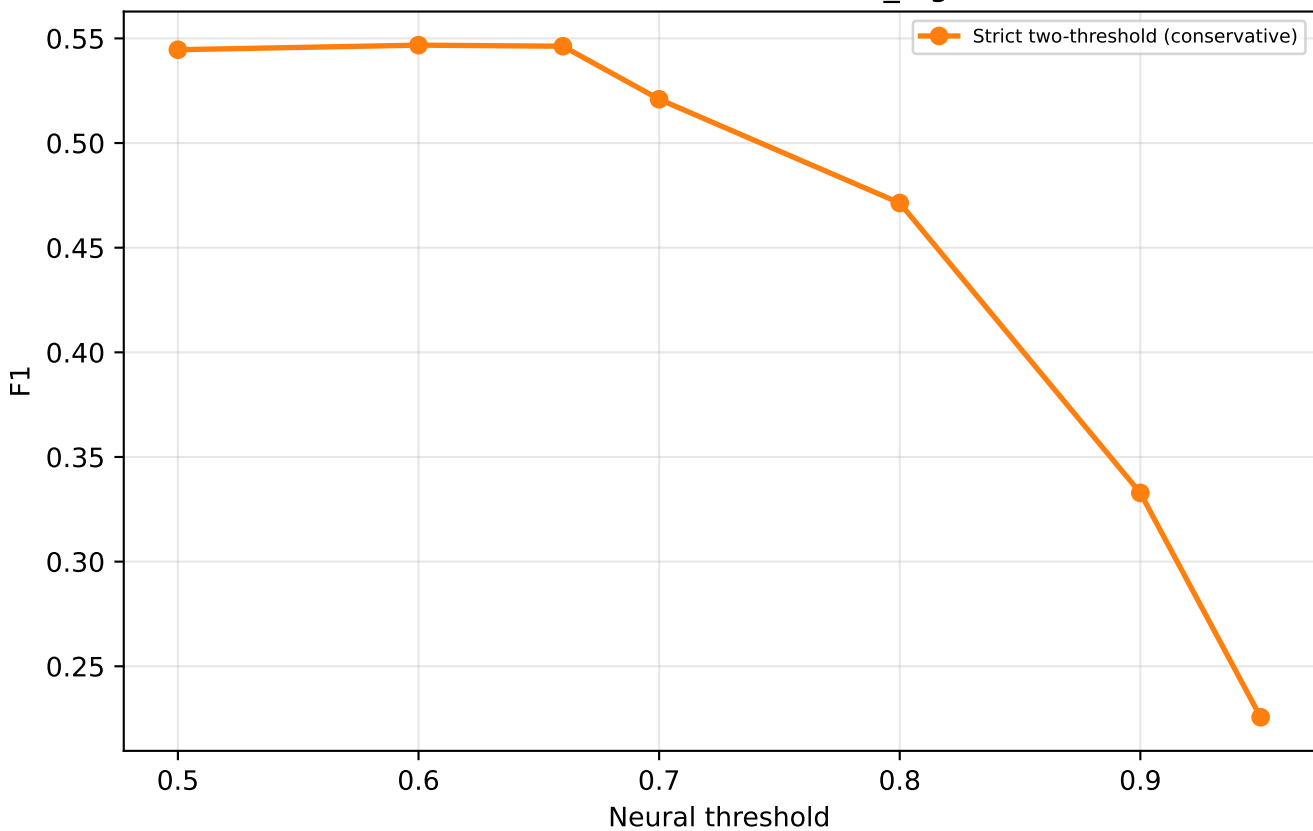
F1 vs threshold — strict conservative \tau_{\text{high}}=0.95 (valid)
