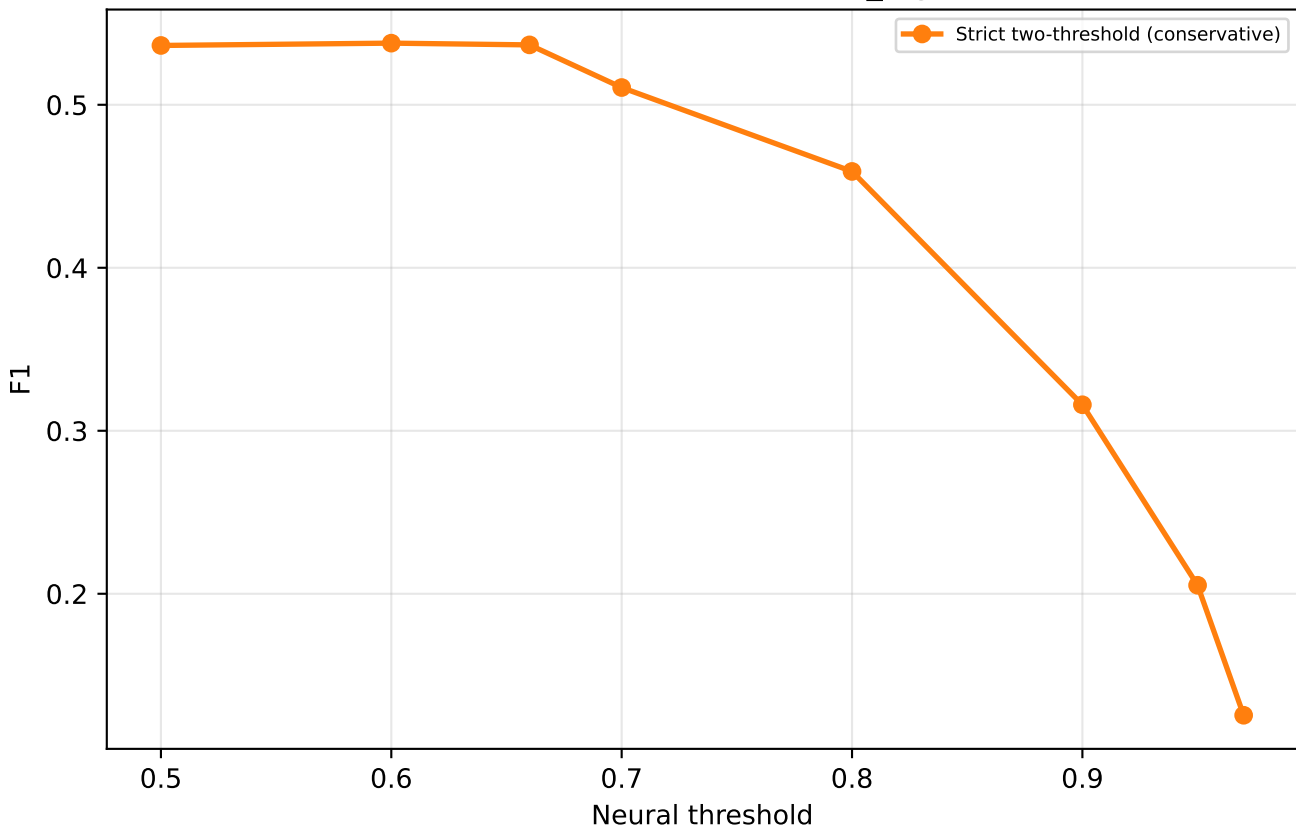
F1 vs threshold — strict conservative \tau_{\text{high}}=0.97 (valid)
