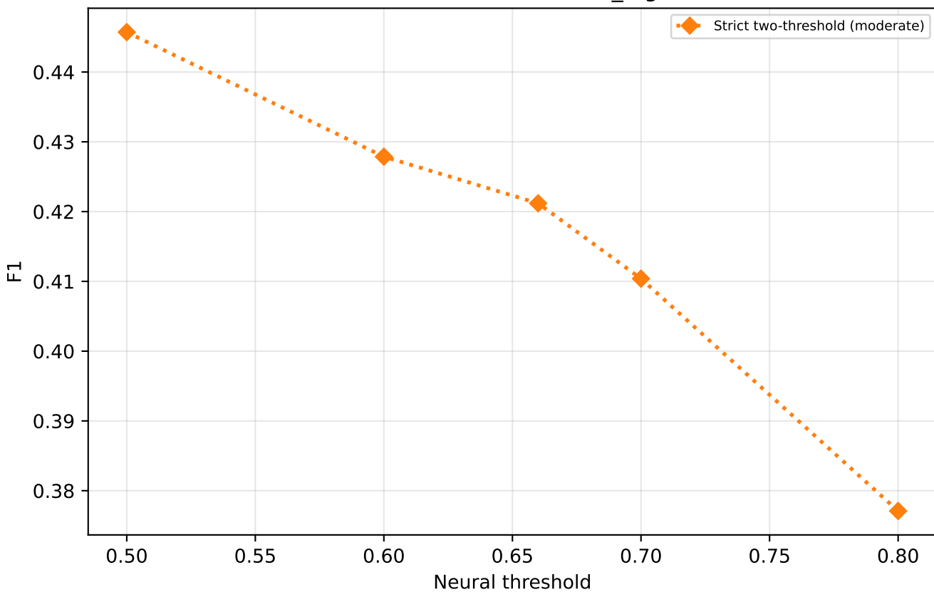
F1 vs threshold — strict moderate \tau_{\text{high}}=0.80 (valid)
