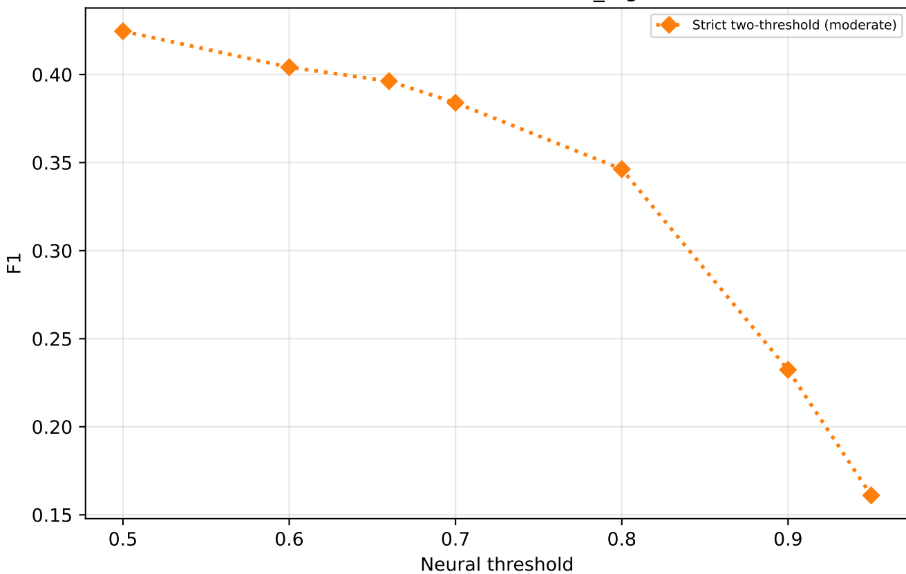
F1 vs threshold — strict moderate \tau_{\text{high}}=0.95 (valid)
