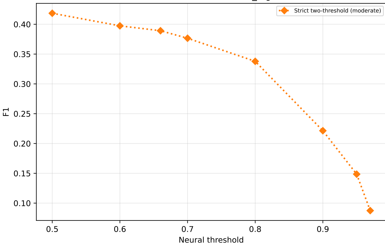
F1 vs threshold — strict moderate \tau_{\text{high}}=0.97 (valid)
