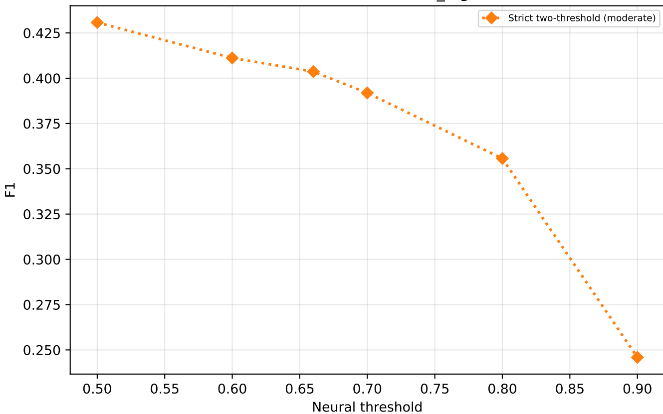
F1 vs threshold — strict moderate \tau_{\text{high}}=0.90 (valid)
