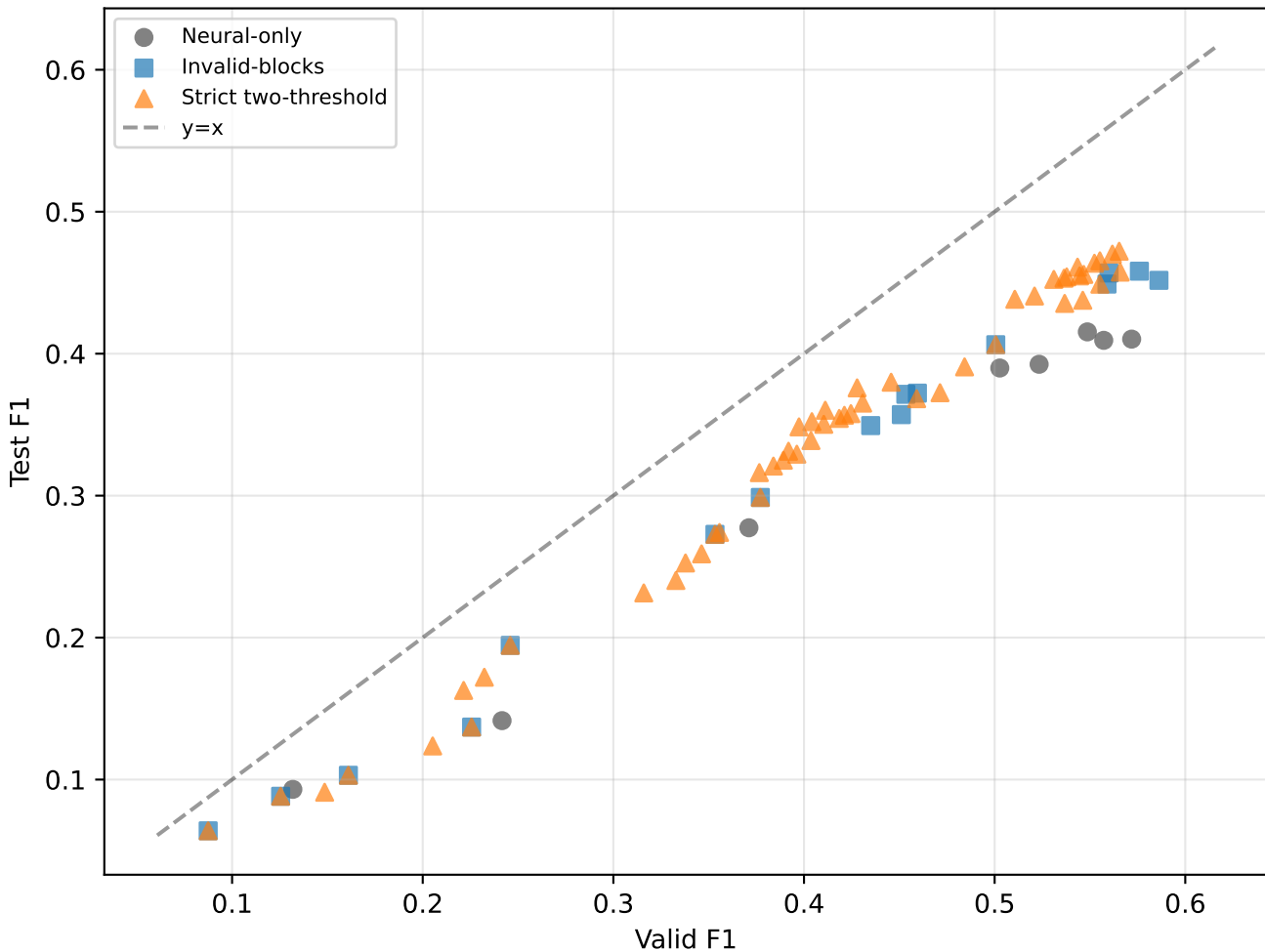
Valid vs test f1
