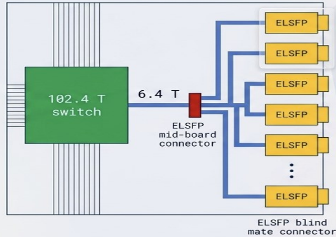
ELSFP (8CH / 20~23 dBm)
