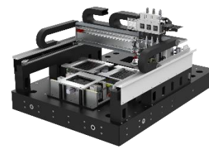
龍門XYZ平台 • 高精度定位
