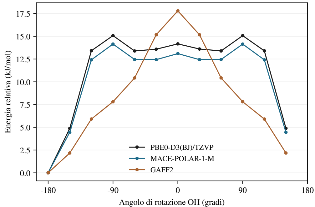
HFIP isolato: geometria fissata salvo H
